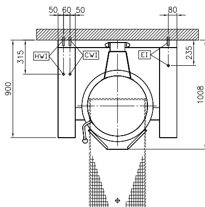
Boven aanzicht
